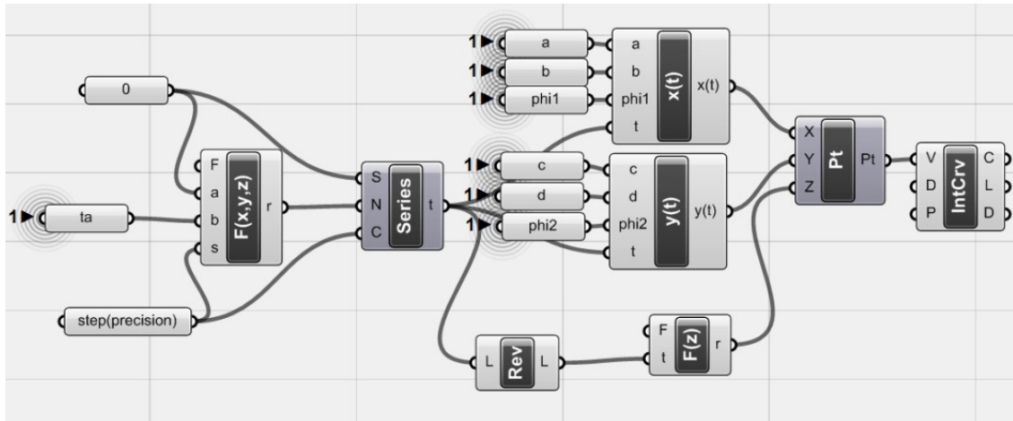
شکل ۱۶: الگوریتم به کار رفته برای ترسیم قطعات منحنی اسپیرال
