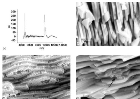
شکل ۷: لایه‌های آراگونیت
