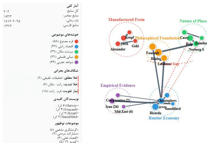
شکل ۱: تحلیلی بیبلومتریک
