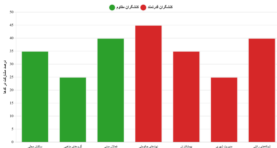
شکل ۵: شبکه کنشگران
